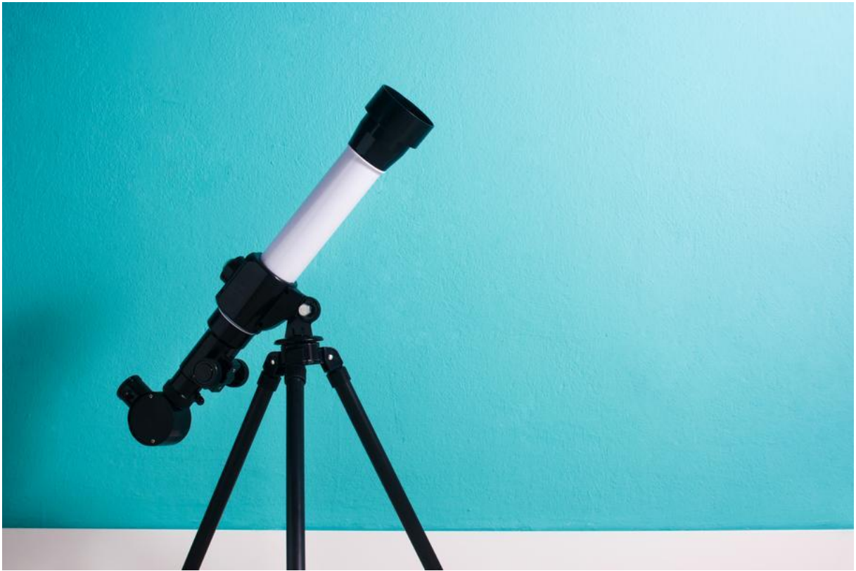
teleskop astronomiczny
