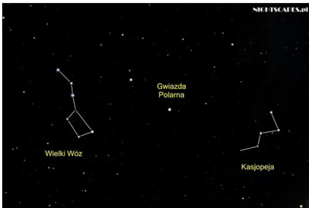
Konstelacja gwiazd
